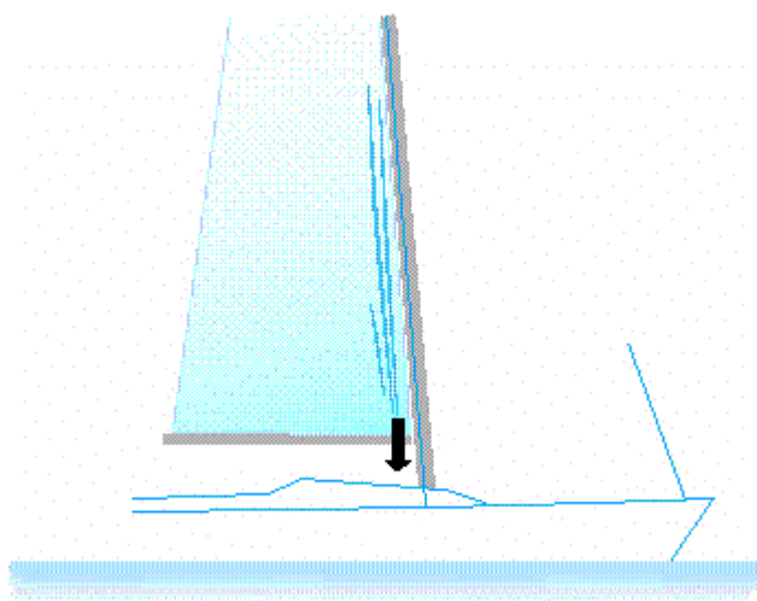
Utan belastning i segelduken bildas ett veck längs mastliket när cunningham sträcks.
