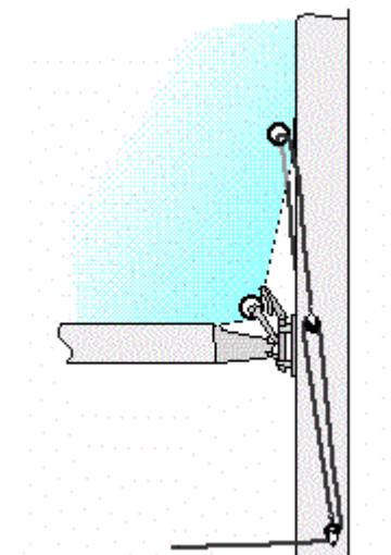
Det är viktigt att cunningham drar något framåt, annars kan travarna eller liklinan ryckas ur seglet. En utväxlad cunningham är alltid lättare att justera
